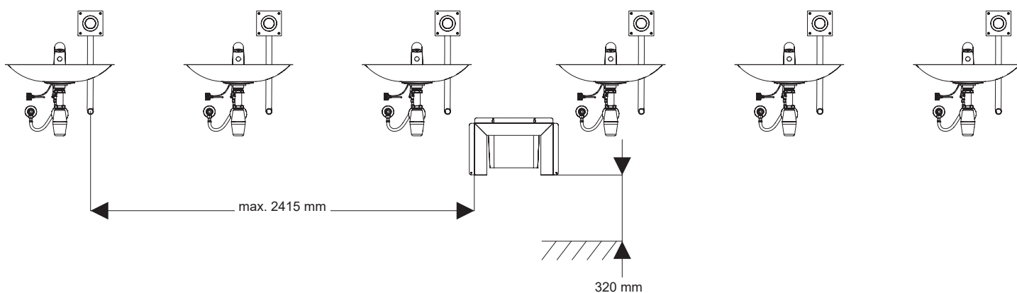
Schéma / Layout
