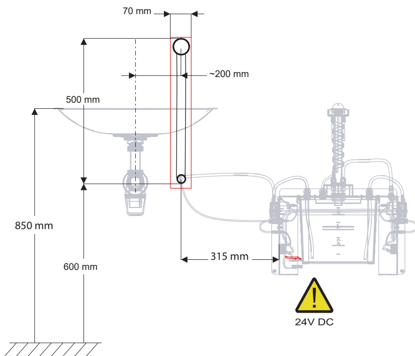
Schéma / Layout
